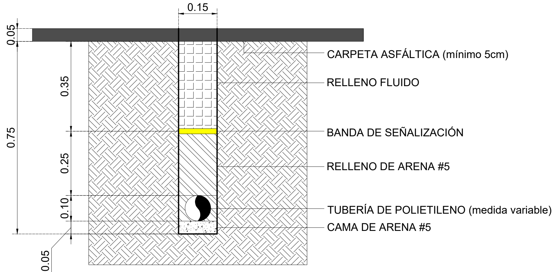
CORTE ESTRUCTURAL (GAS)
